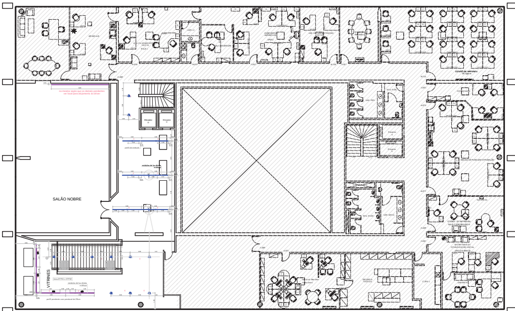
1 PLANTA BAIXA - 2º PAVIMENTO
